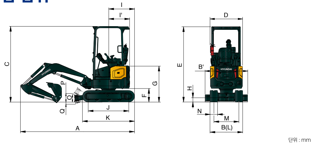
단위 : mm
