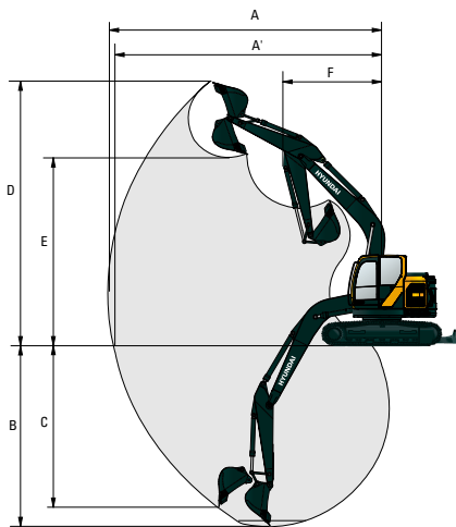
작업범위 (단위 mm)
